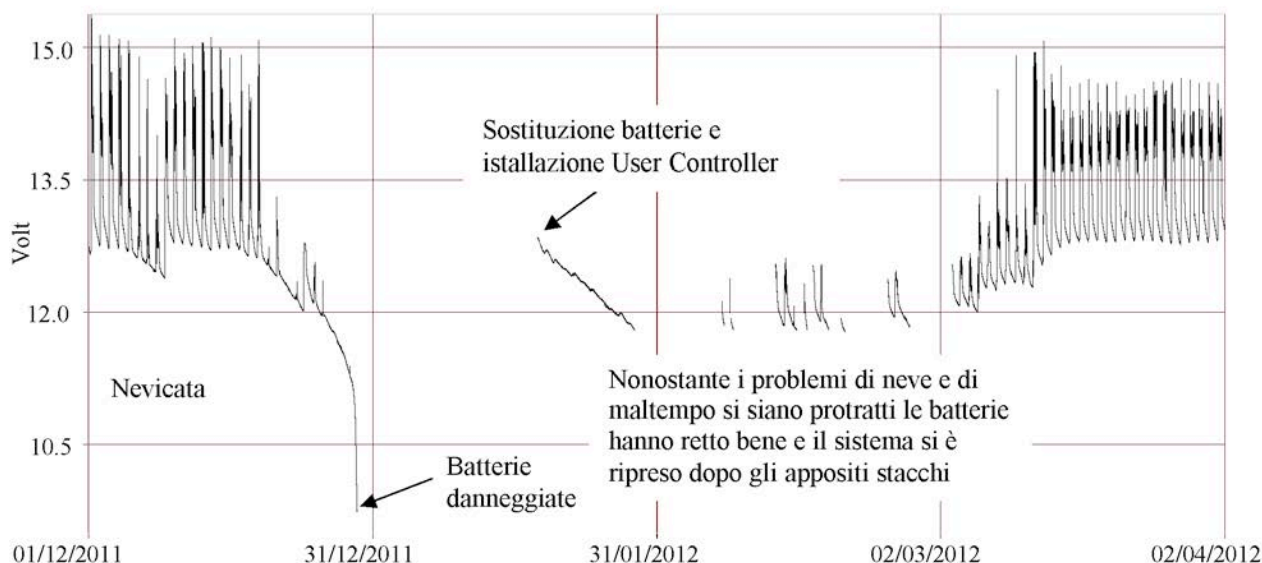
Figura 10. Tensione di batteria registrata alla stazione dilatometrica di M.te Egitto. Nel periodo invernale l'utente controller è intervenuto più volte con appositi stacchi a salvaguardare le batterie, che si sono regolarmente riprese quando il tempo atmosferico è migliorato.
