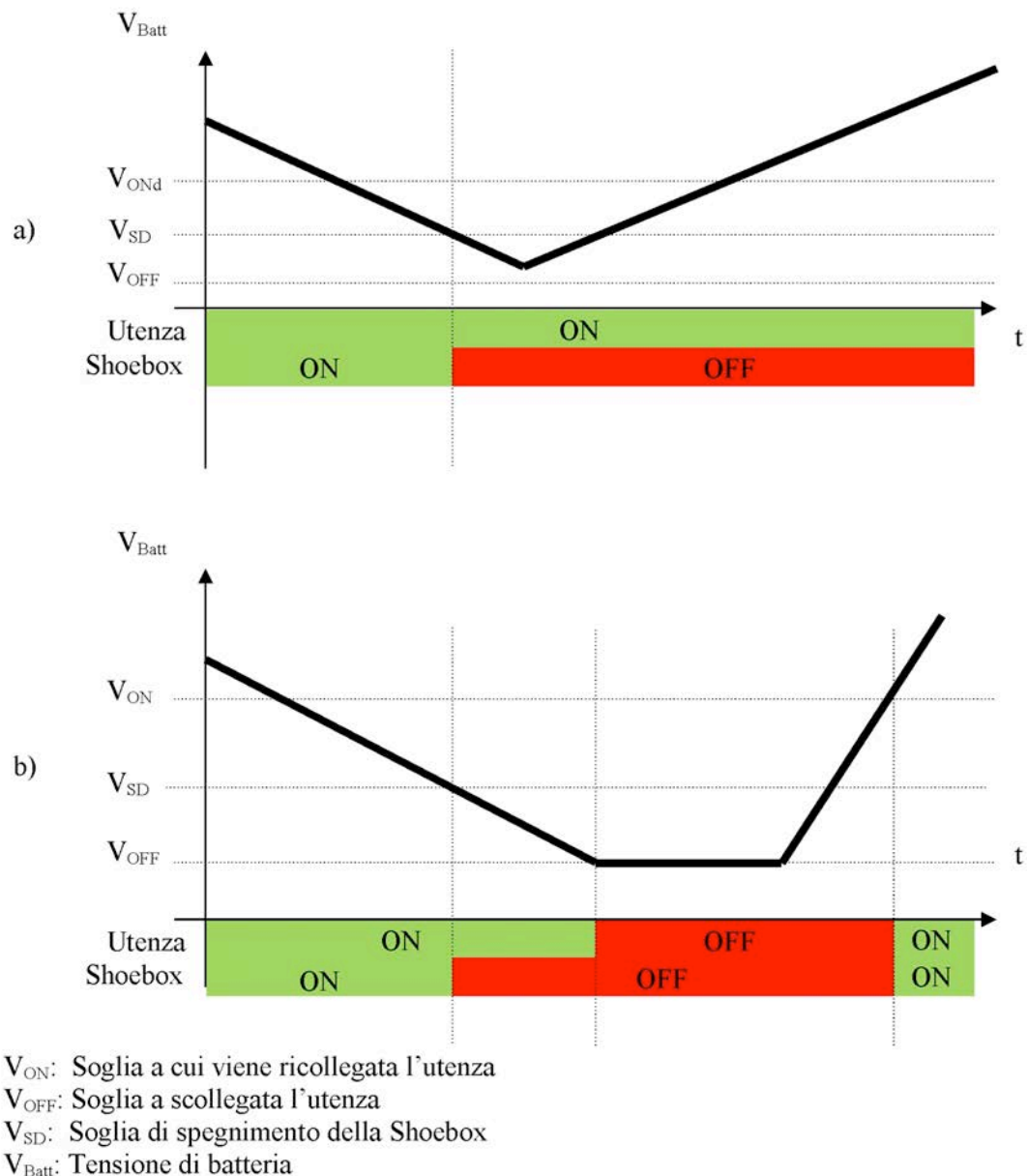
Figura 7. Timing del distacco energetico: a) la Shoobox esegue lo shutdown su un falso segnale e rimane spenta indefinitamente; b) la Shoobox esegue lo shutdown e si riaccende normalmente quando l'utenza viene ricollegata.
