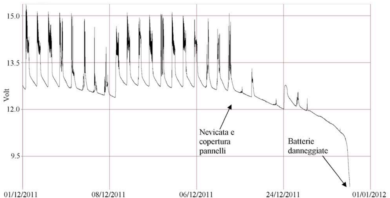
Figura 6. Tensione di batteria campionata alla stazione dilatometrica di M.te Egitto.
