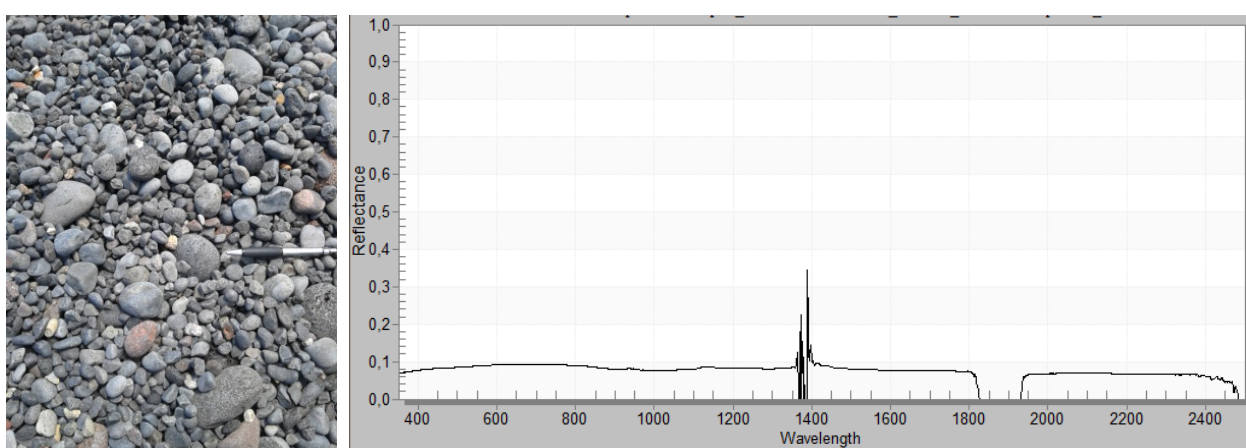
Figura 14. Esempio di una firma spettrale al ciottolato presso la spiaggia di Acquacalda.
