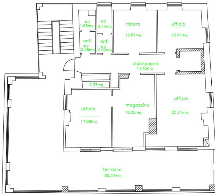
Piano terra - rialzato
